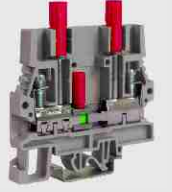
SCB.6/DD/GR (6mm 2 ayırma klemensi)
