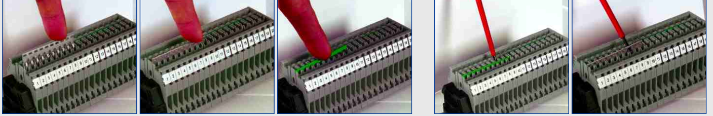
Geçmeli Tip Üst Köprü Montajı ve Sökülmesi
